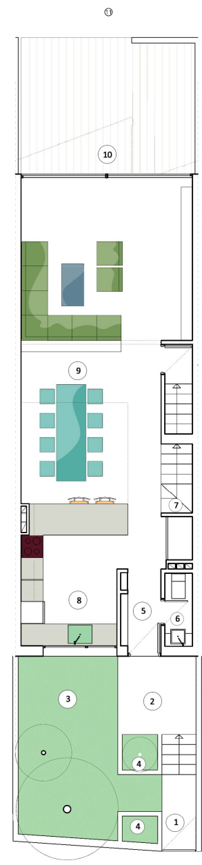
planta baja
